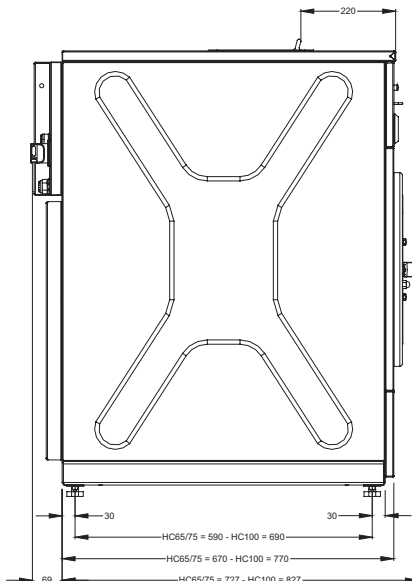
zij aanzicht HC 65-75-100
