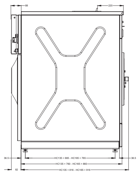
zij aanzicht HC 135-165
