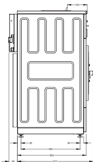
zij aanzicht HC 60
